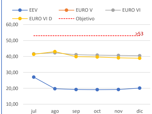
Consumo l/100 km por tipo de vehículo
