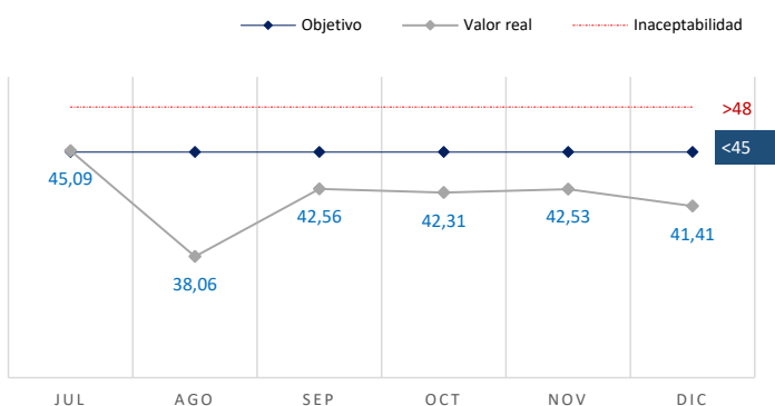
Consumo de combustible en las unidades (l)/100km
