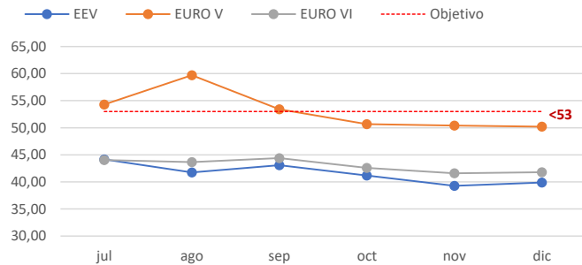
Consumo l/100 km por tipo de vehículo
