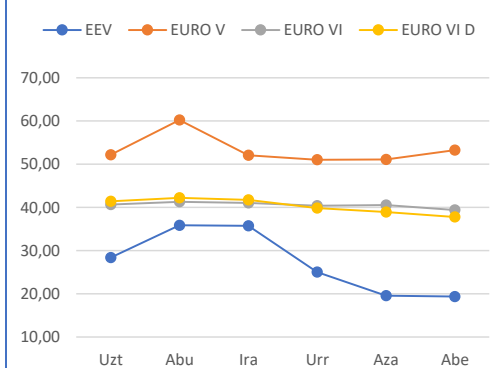
Consumo l/100 km por tipo de vehículo
