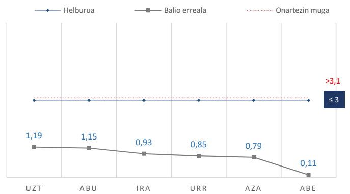
Hilean unitateen/bidaiariaren kW-aren kontsumoa
