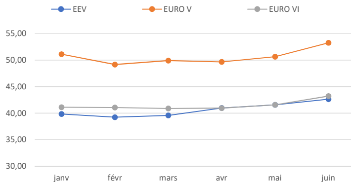
Consommation l/100 km par type de véhicule
