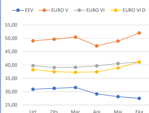
kontsumoa litrotan 100 kilometroko teknologien sailkapenaren arabera
