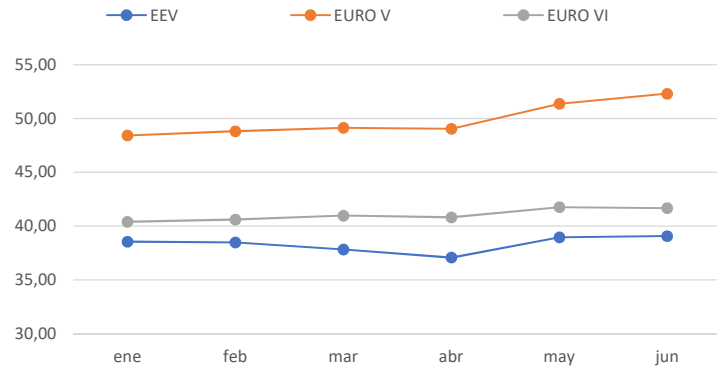
Consumo l/100 km por tipo de vehículo
